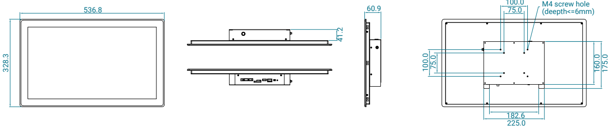
GPC-C215MB
