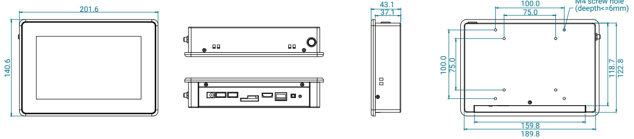
GPC-C070MB
